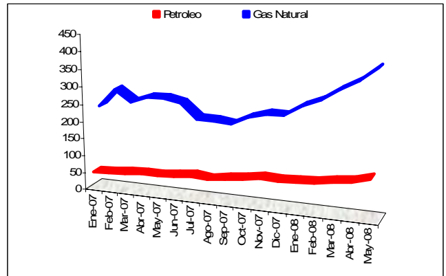
Precio del Petróleo y Gas Natural (Gas Natural: dólares por mil metros cúbicos / Petróleo: dólares por barril)
